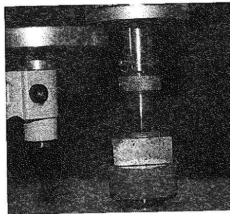
รูปที่ 2 แสดงการทดสอบค่ากำลังแรงยึดด้วยเครื่องทดสอบเอนกประสงค์ชนิดอินสตรอน รุ่น 8872 ด้วยหัวกดรูปทรงกระบอกที่มีขนาดเส้นผ่าศูนย์กลาง 0.8 มิลลิเมตร
